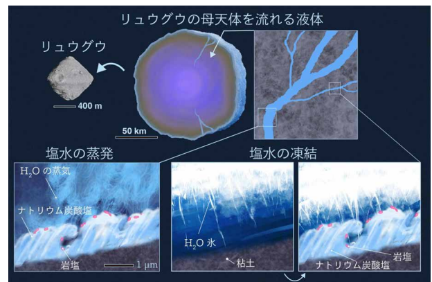
図4 リュウグウの母天体での塩結晶の形成過程
