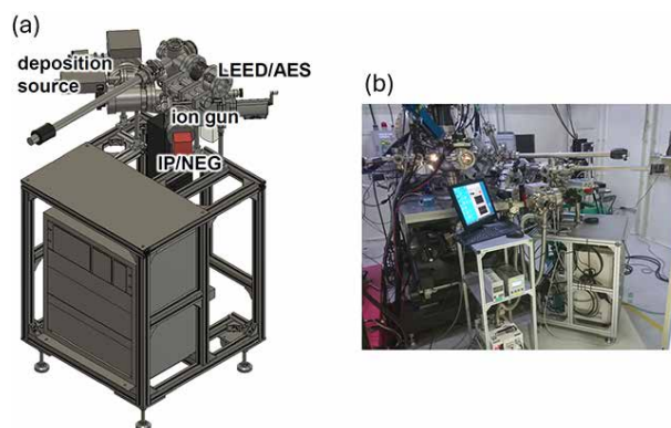
図3 (a) 可搬式試料準備チェンバーの概略図 (b) BL09XU EH2 3次元空間分解 HAXPES 装置への接続時の写真
