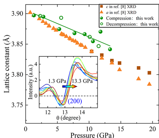
図4 200面のKossel線から求めた格子定数の圧力変化。挿入図はKossel線のプロファイルを示す [8] 。
