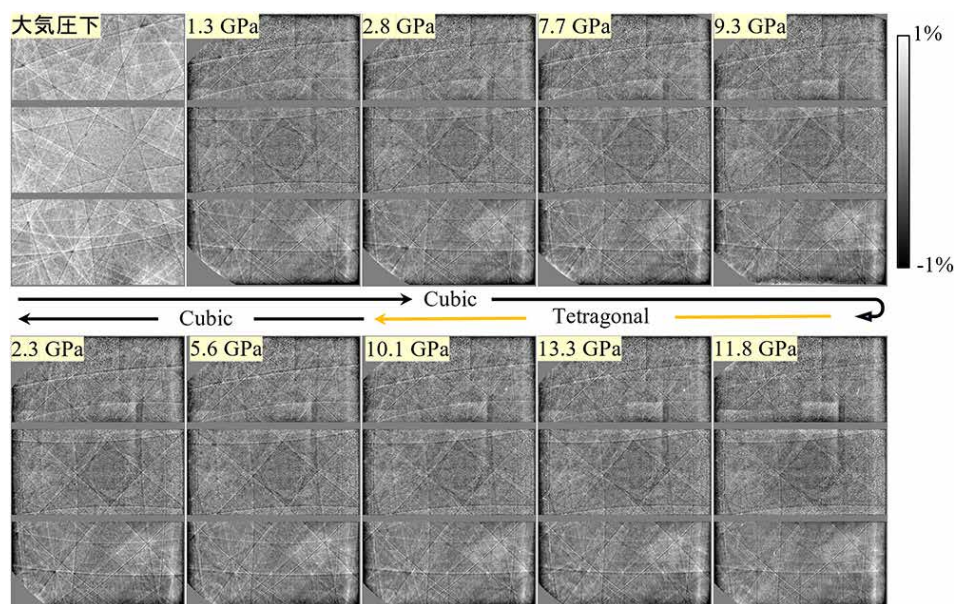
図3 DAC中のSrTiO 3 単結晶試料から得られた高圧下ホログラム像の圧力変化。左上の大気圧下のXFH像はDACなしで測定された。
