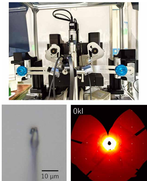
図2 微小結晶ハンドリングシステムの外観(上)、ピックアップした結晶の写真(左)、および擬プリセクションイメージ(右)
