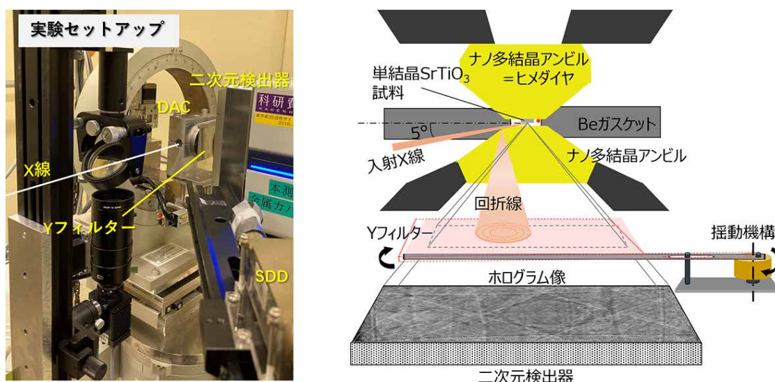
図1 実験のセットアップの写真とダイヤモンドアンビルセル（DAC）まわりの実験配置の模式図。
