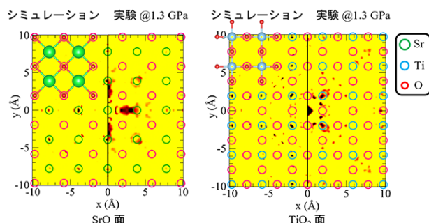
図5 高圧下XFH像から再生されたSrTiO 3 の原子像。
