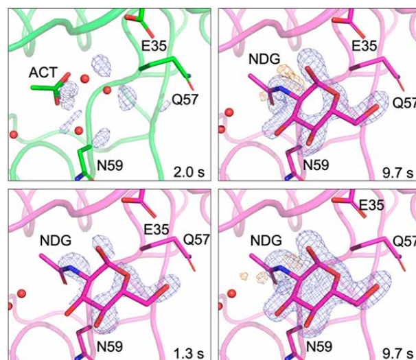
図3 リゾチームに結合する阻害剤の電子密度の変化 リゾチームの活性部位構造の主鎖(線)を主に表示している。一部のアミノ酸残基の側鎖は棒モデルにて表示している。上段は3~5 μm結晶を用いた実験結果、下段は1 μm結晶を用いた結果。右下の数字はそれぞれ混合時間を意味する。2.0 s: 緑で描画されている図は、炭素原子(Cα)を繋いだ主鎖構造を意味する。赤は酸素原子、青は窒素原子を意味し、赤で表示した球は水分子である。青色のメッシュは差フーリエマップ( F_o(\text{混合後}) - F_o(\text{混合前}) )を表す(上二つは5σ、下二つは6σで描画)。ACTは酢酸イオン、E35、Q57、N59はアミノ酸残基(一文字表記)である。ピンク色で表示された図はピンク色が炭素原子を意味し、酸素原子と窒素原子はそれぞれ赤、青である。NDGは阻害剤を意味する。
