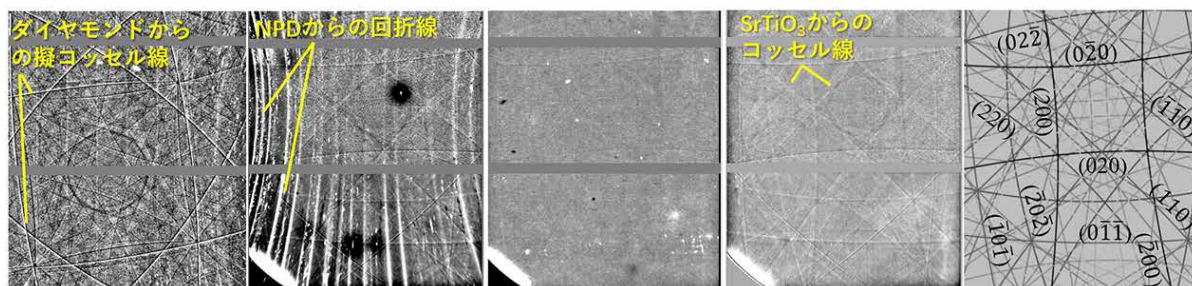
図2 DAC中のSrTiO 3 単結晶試料から得られた高圧下ホログラム像のノイズ除去のプロセス。NPDアンビルと揺動するYフィルターによって、高圧下でもSrTiO 3 試料の単結晶性に由来するKossel線を含む明瞭なホログラム像が得られた。
